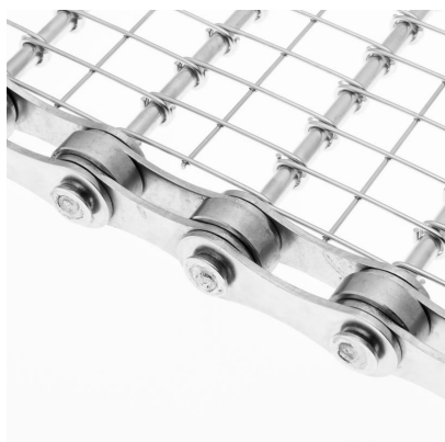
Tapis métallique avec des tiges électro-soudées et de chain latéral
